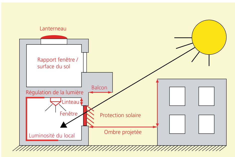
Illustration 35: Facteurs d'influence de l'utilisation de la lumière du jour se- lon la norme SIA 380/4.
