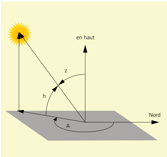
Illustration 146: Diagramme standard solaire polaire pour la latitude 51^\circ\text{N} (Cologne, Erfurt, Dresde)
