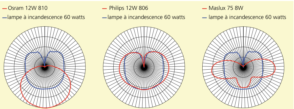
Illustration 84: Répartition de la lumière des lampes Retrofit sélectionnées (rouge = LED, bleu = lampe à incandescence 60 watts).
