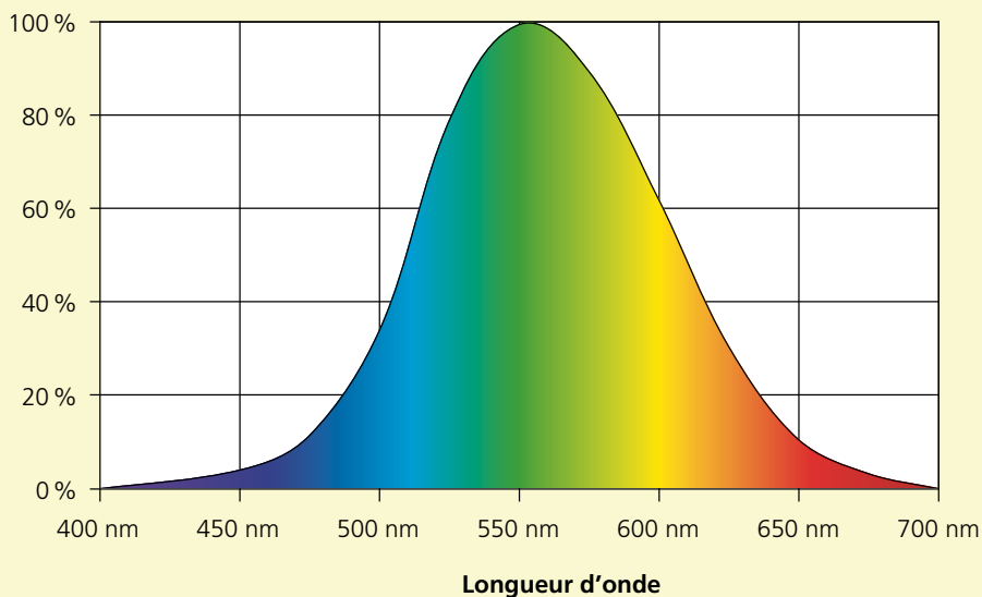
Illustration 17: Sensibilité de l'œil humain selon le spectre visible (courbe V-lambda).
