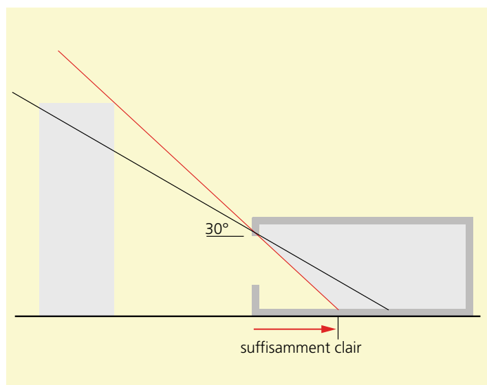
Illustration 151: La règle des 30° de lucarne.
