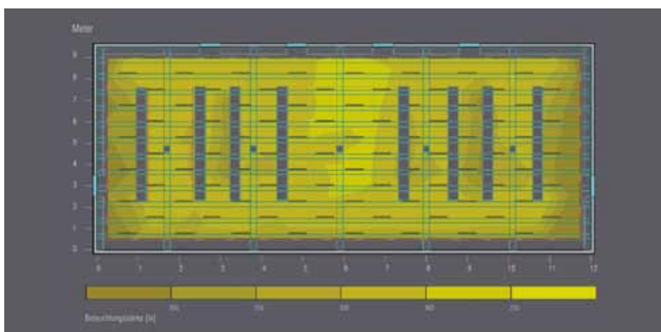
Illustration 180: Répartition de l'éclairage lumi- neux (bibliothèque can- tonale, Liestal).
