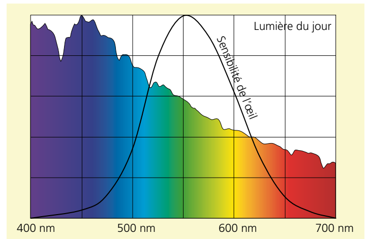
Illustration 75: Spectre visible d'une lampe à incandescence.
