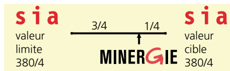
Illustration 41: Définition des exigences Minergie pour l'éclairage entre valeur limite et valeur cible.
