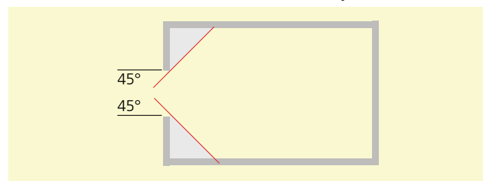
Illustration 153: Définition du facteur de lumière du jour.
