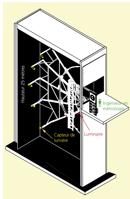
Illustration 100: Principe d'un photogoniomètre avec mouvement de la tête du photomètre (Zumtobel, Dornbirn).
