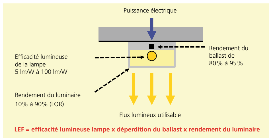
Illustration 102: Définition du facteur d'efficacité des luminaires LEF.
