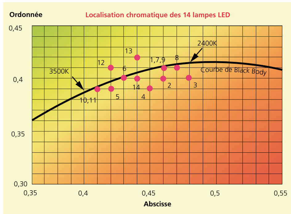
Illustration 83: Localisation chromatique des 14 lampes LED Retrofit mesurées (extrait du triangle des couleurs).
