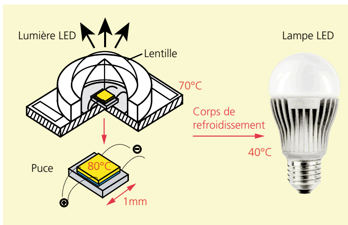
Illustration 73: La gestion thermique et la qualité de l'appareil déterminent la durée de vie.
