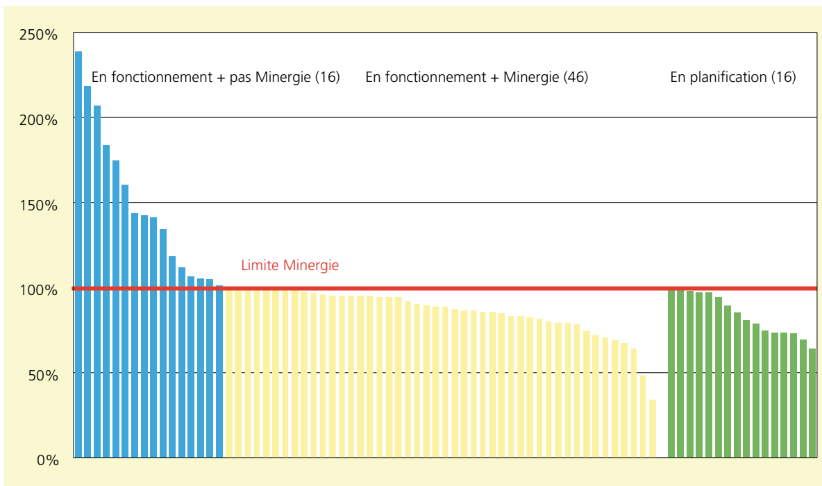
Illustration 52: Contrôle Minergie systématique des éclairages dans les bâtiments propriété de la ville de Zurich.
