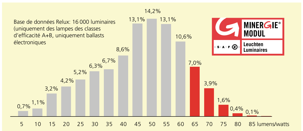
Illustration 42: Interprétation de la base de données Relux selon les facteurs d'efficacité des luminaires.
