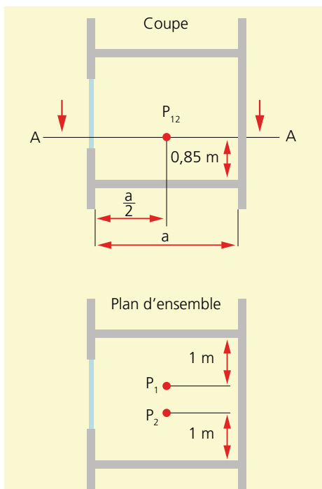
Illustration 149: Points de référence pour la définition de la luminosité suffisante selon DIN 5034-1 pour les ouvertures latérales.
