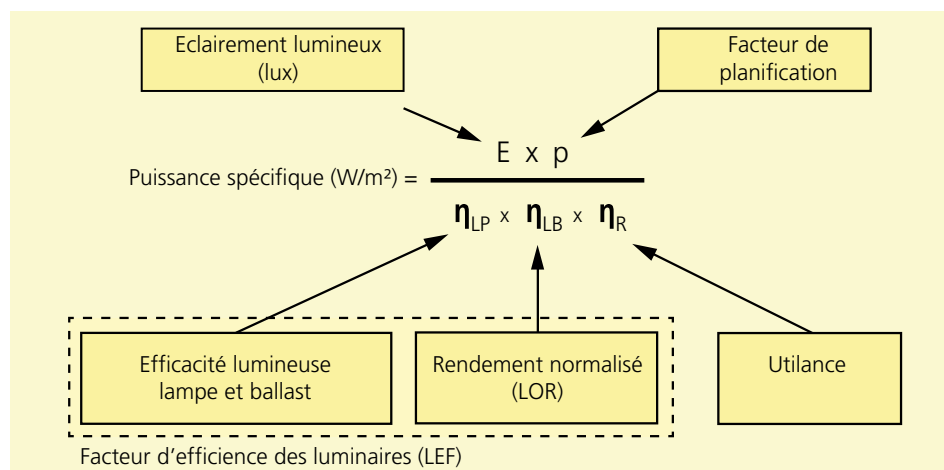
Illustration 32: Calcul de la puissance installée selon la norme SIA 380/4.
