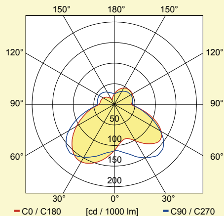
Illustration 99: Luminaire de bureau
