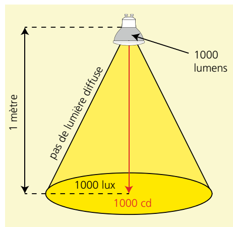
Illustration 19: Relation entre l’éclairage lumi- neux (lux), le flux lumineux (lumens) et l’intensité lumi- neuse (candela) dans le cas d’une lu- mière dirigée.
