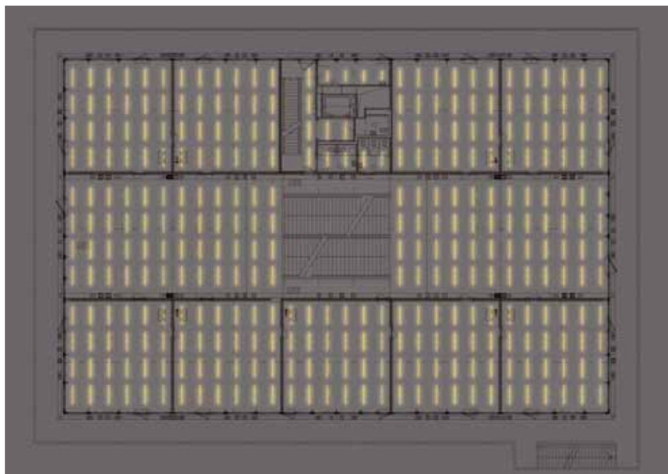
Illustration 162: Plan d'ensemble 1 er étage, bâtiment scolaire Leutschen- bach, avec les posi- tions des lumi- naires.
