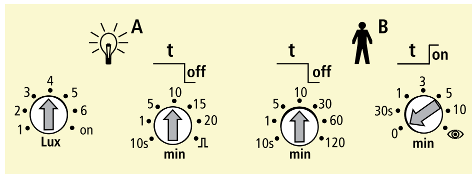
Illustration 113: Schéma de réglage en combinaison avec un capteur de présence-lumière du jour (HTS Theben).
