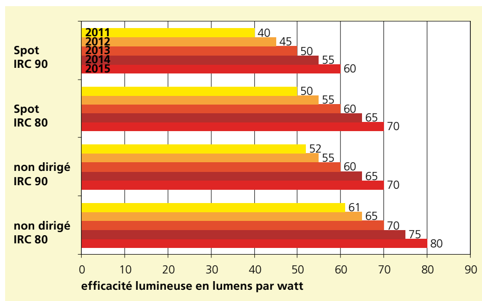
Illustration 85: Exigences posées aux lampes LED-Re- etrofit selon la charge de qualité UE (IRC: Index de rendu des couleurs).
