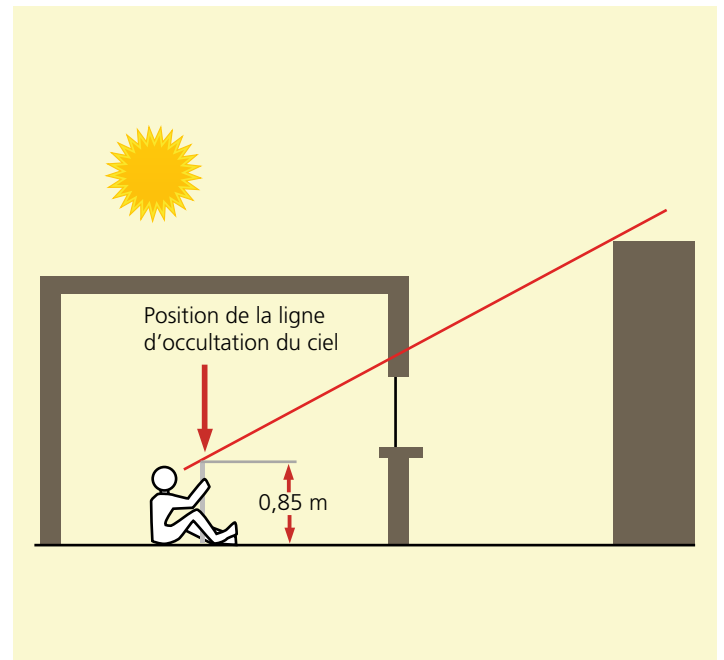
Illustration 148: Règle des 30^\circ .
