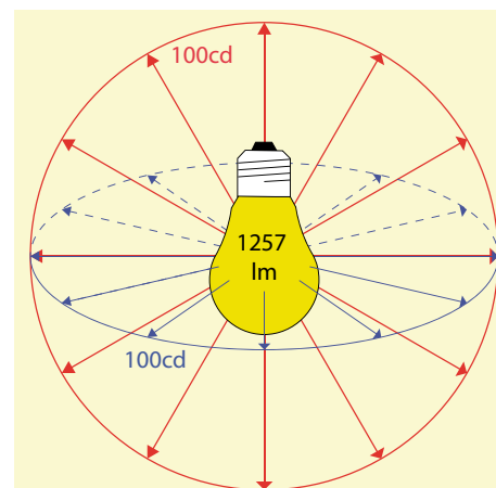
Illustration 20: Relation entre lu- men et candela dans le cas d’une lu- mière à rayonne- ment uniforme.
