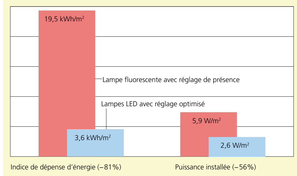
Illustration 124: 56% d'économie de la puissance installée et 81% d'économie de la consommation d'énergie.
