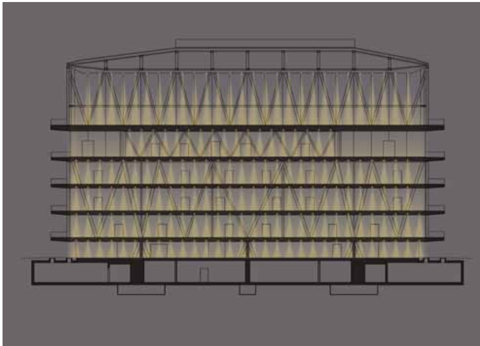
Illustration 161: Coupe à travers le bâtiment scolaire Leutschenbach.
