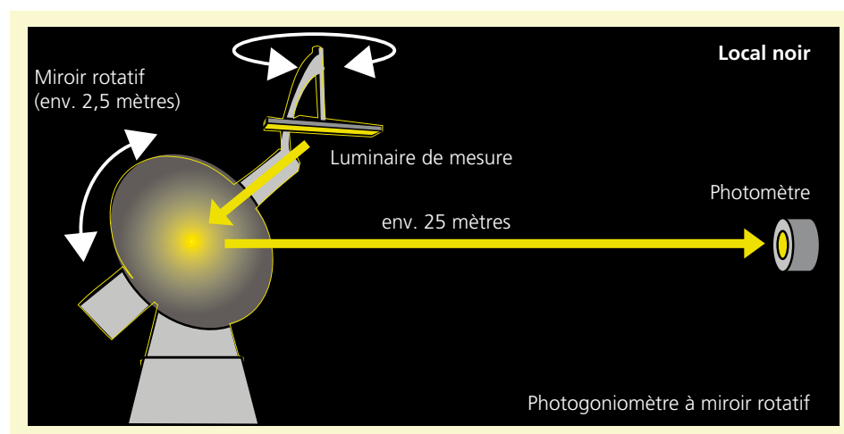
Illustration 101: Principe d'un photogoniomètre à miroir rotatif (Metas Berne).
