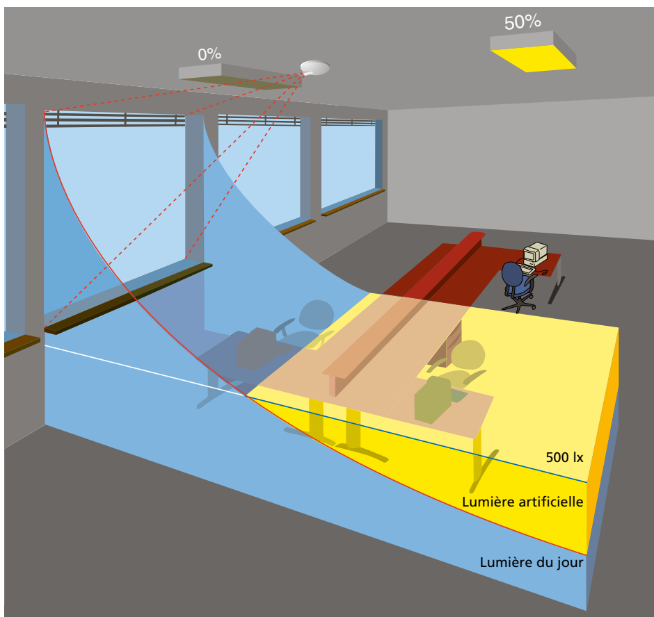
Illustration 144: Représentation schématique d'un réglage de la luminosité constante.
