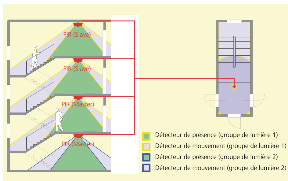
Illustration 111: Exemple de planification PIR dans une cage d'escalier (Swisslux).
