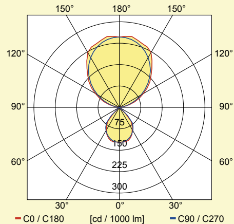
Illustration 96: Luminaire sur pied
