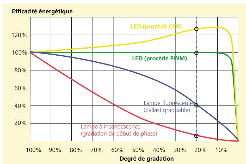
Illustration 69: Efficacité énergétique en relation avec le degré de gradabilité des lampes LED en comparaison avec les lampes fluorescentes et les lampes à incandescence.
