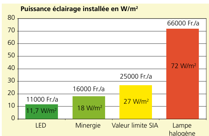
Illustration 198: Comparaison de la puissance installée de l'éclairage et des coûts de l'électricité dans le supermarché (en Fr. par an).
