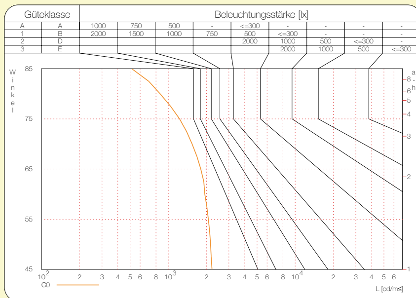
Illustration 39: Procédé de courbes limites selon Söllner (Diagramme de Söllner).
