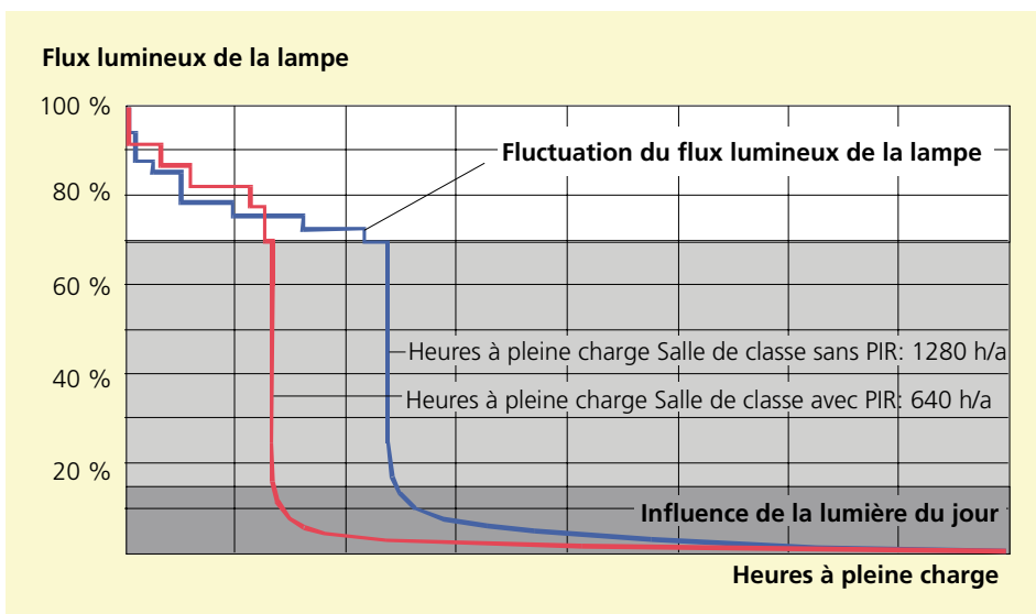
Illustration 119: Mesure des heures à pleine charge pour l'éclairage dans deux salles de classes, avec et sans détecteur de présence.
