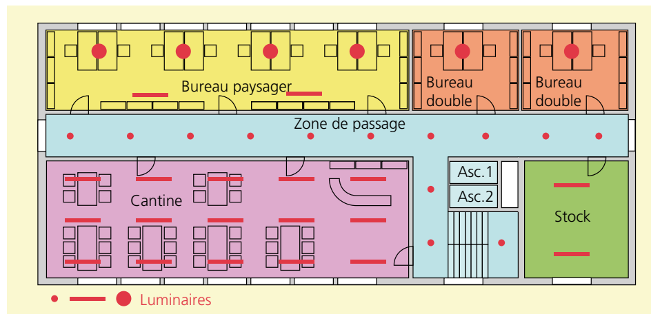
Illustration 37: étage typique d'un bâtiment, différencié selon les utilisations.
