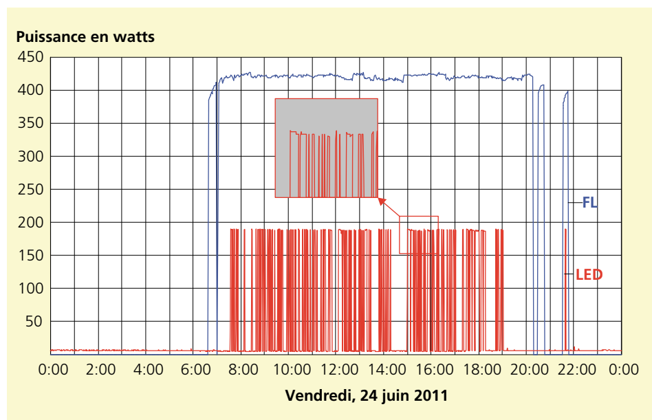
Illustration 123: Courbe journalière de la puissance lors d'une journée de travail usuelle; le couloir à LED consomme 81% d'énergie de moins que le couloir avec lampes fluorescentes.
