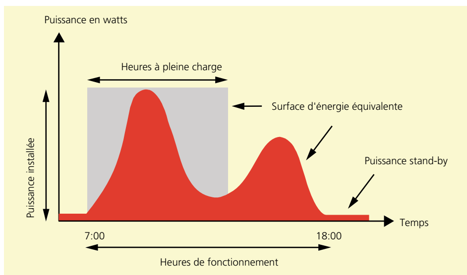
Illustration 29: Définition des heures à pleine charge.
