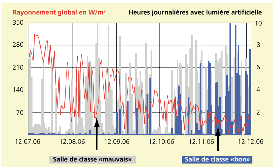
Illustration 118: Variation annuelle du rayonnement global et des heures de fonctionnement de l'éclairage artificiel dans deux salles de classe différentes avec une commande dépendant de la lumière du jour et de la présence.
