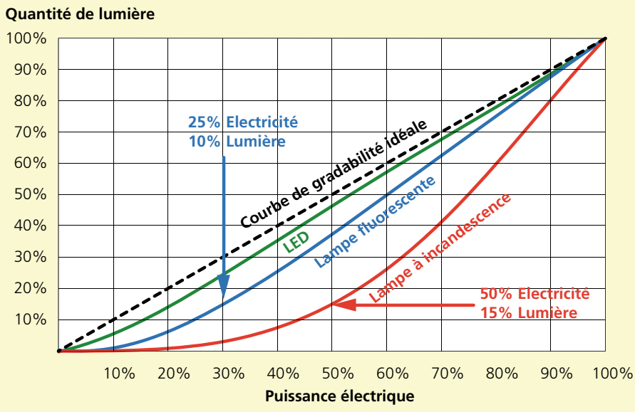
Illustration 62: Comportement de gradabilité des trois types de lampe.
