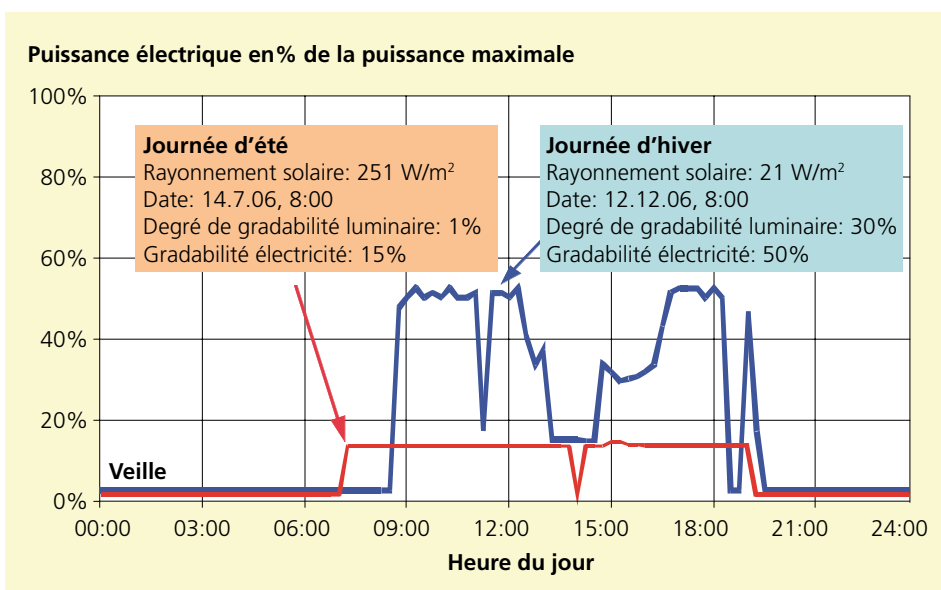
Illustration 120: Profil journalier de la puissance électrique en cas de réglage de la luminosité constante.
