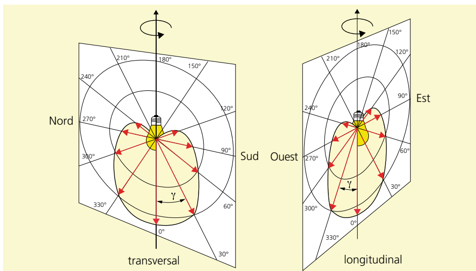
Illustration 15: Courbe de répartition de la lumière d'une lampe à incandescence dans le sens longitudinal et transversal.
