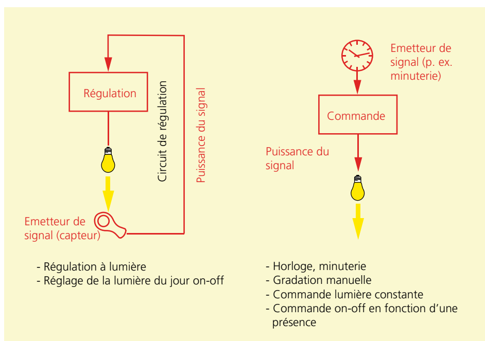
Illustration 106: Différence entre régulation et commande.
