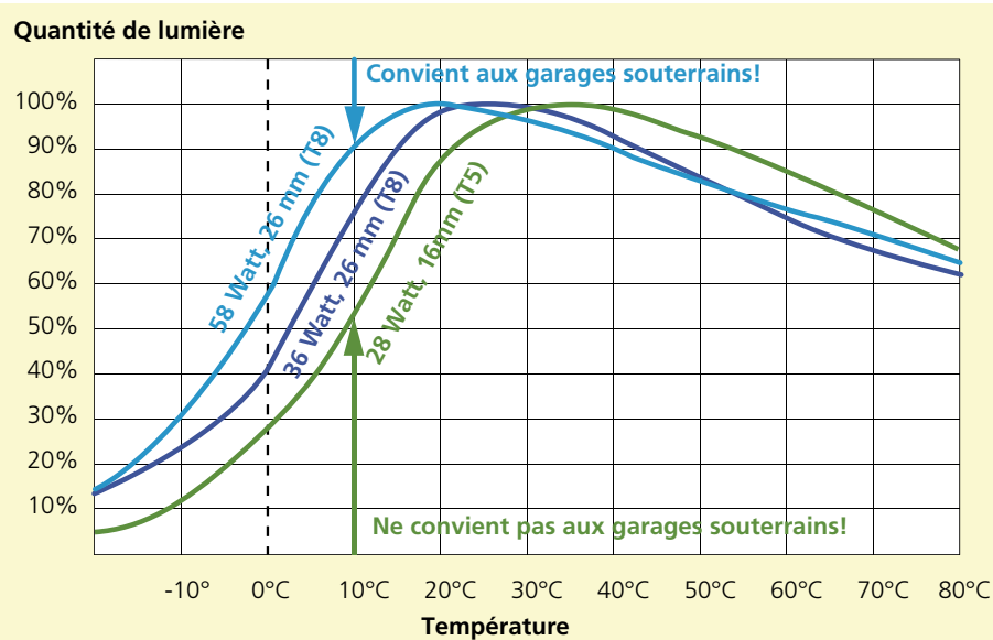
Illustration 63: Quantité de lumière dépendante de la température dans les lampes fluorescentes.
