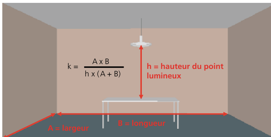
Illustration 30: Définition de l'indice du local.
