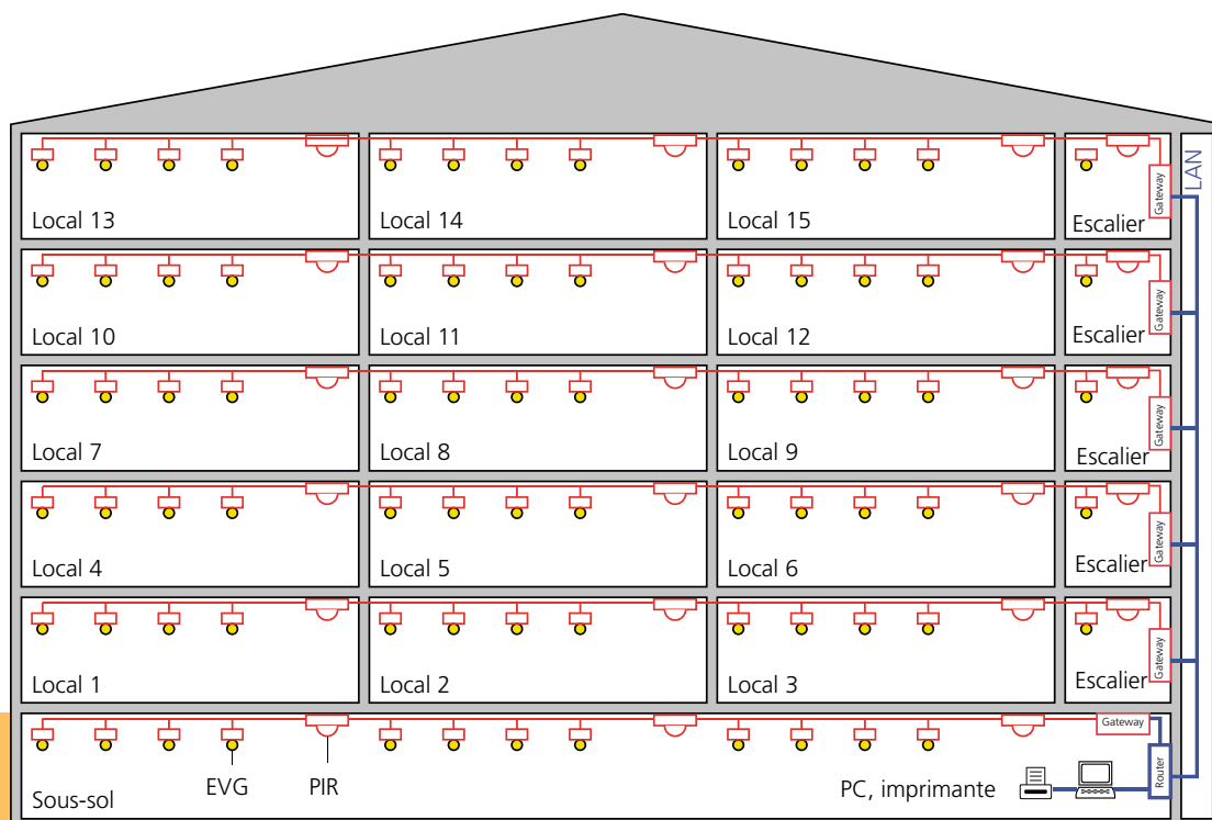
Illustration 116: Composants de la gestion de la lumière.
