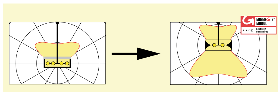
Illustration 156: Répartition de la lumière non idéale et optimale.
